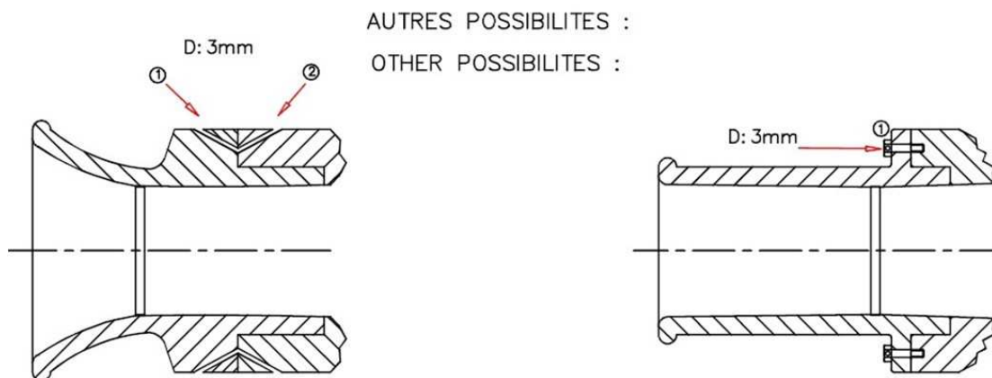
DIBUJO TECNICO Nº 2 ESQUEMA DE TURBO PARA PRECINTAJE DE TODOS LOS
