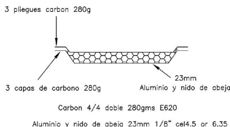
Dibujo N°255-14
