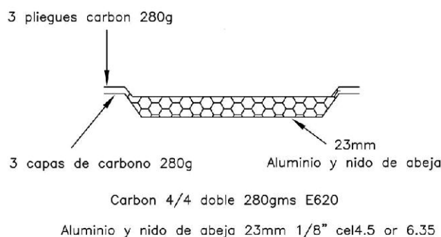
Dibujo N°255-14
