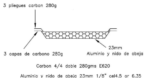
Dibujo N°255-14
